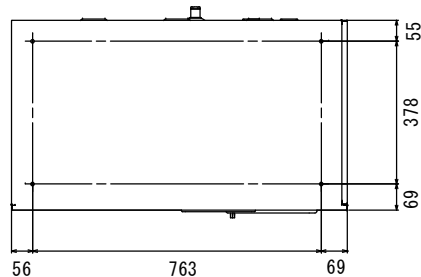
【底面開口部】
